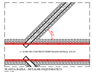
PLANTA BAIXA - DETALHE ESQUEMÁTICO ESC: 1/20
