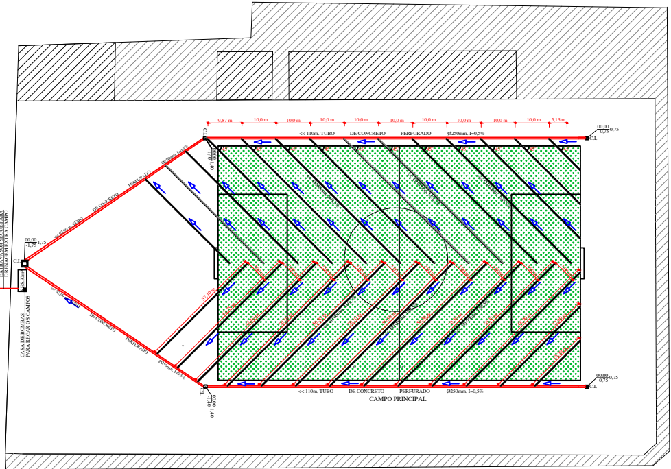
PLANTA BAIXA - DRENAGEM ESC: 1/500
