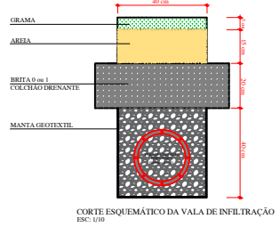
CORTE ESQUEMÁTICO DA VALA DE INFILTRAÇÃO ESC: 1/10
