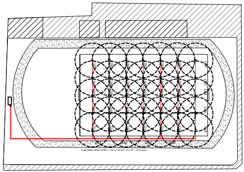
PLANTA BAIXA - IRRIGAÇÃO ESC: 1/1000
