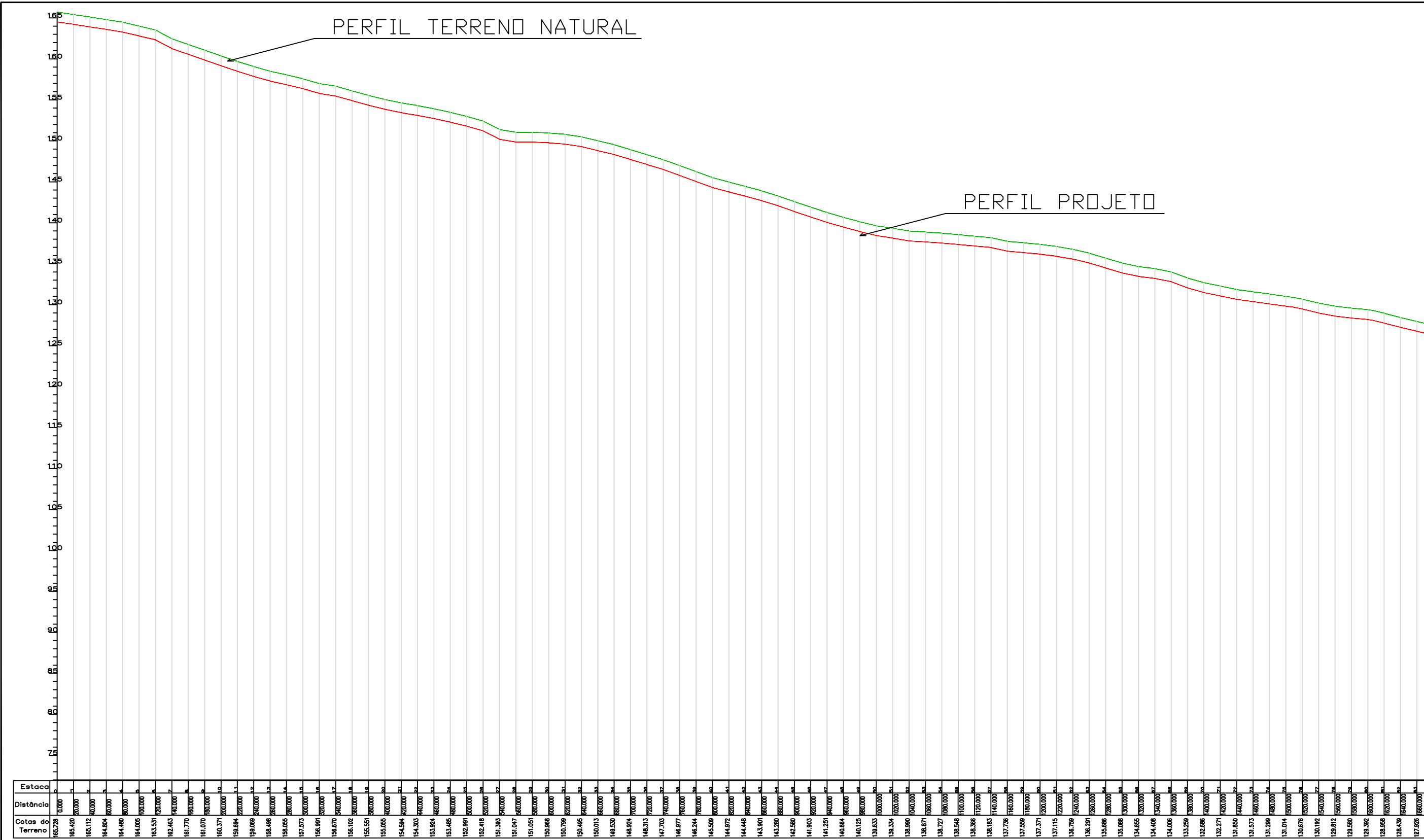
PERFIL LONGITUDINAL RAMAL PRINCIPAL (ADUTORA)
